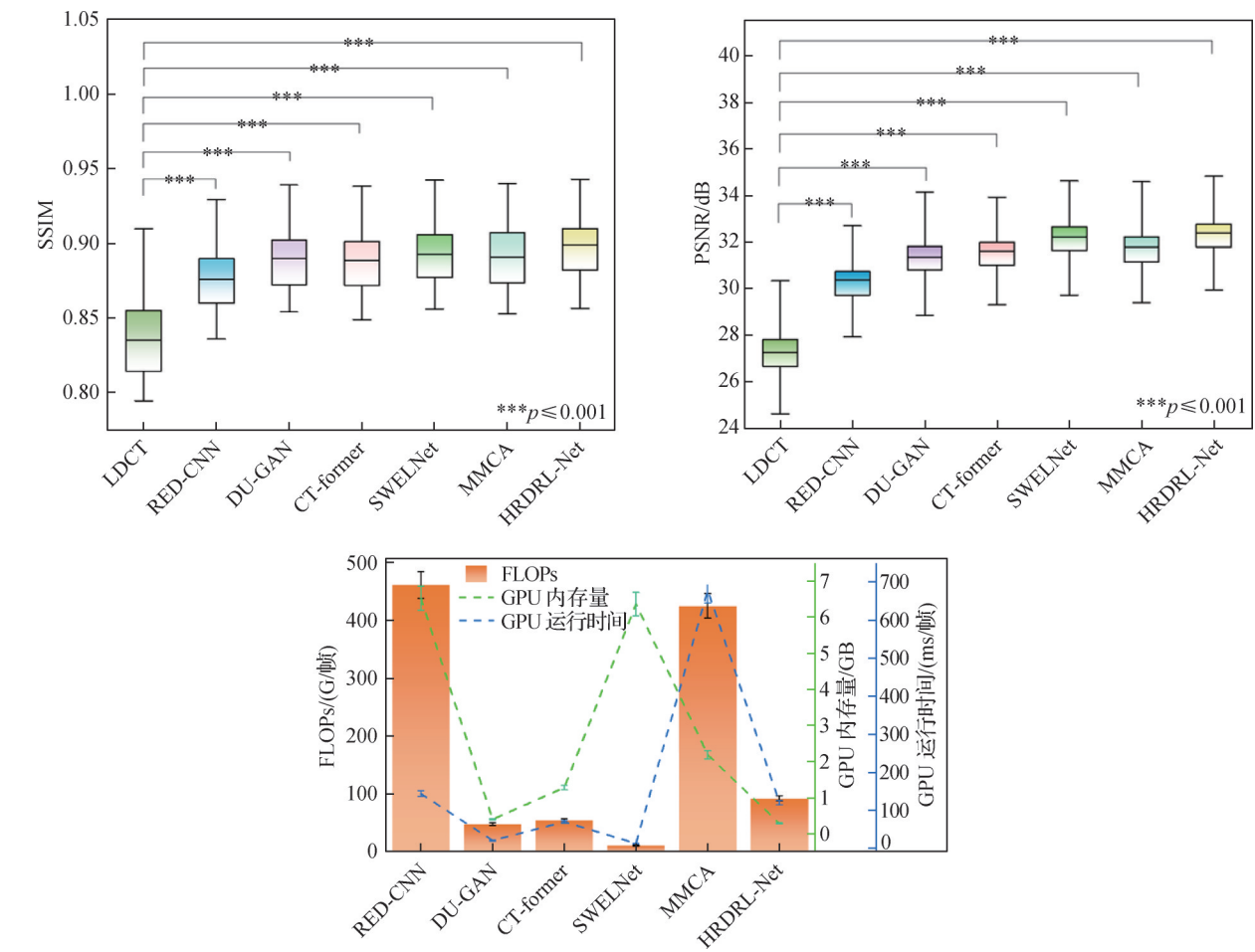
图8 对 Mayo 测试集中全部样本进行图像重建的评价指标统计结果
