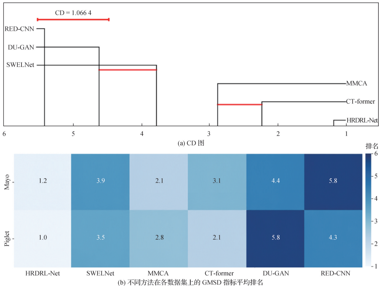
图 11 Friedman 检验结果
